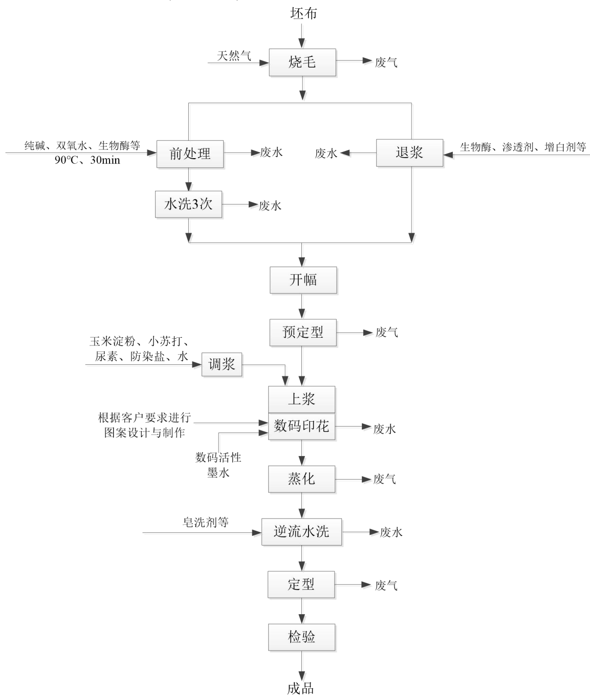
图 2.2-1 人棉机织布印花(数码印花)生产工艺流程图
