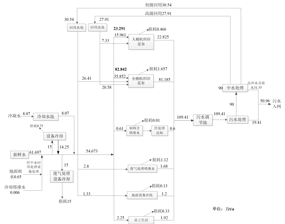
图 2.1-1 项目水平衡图
