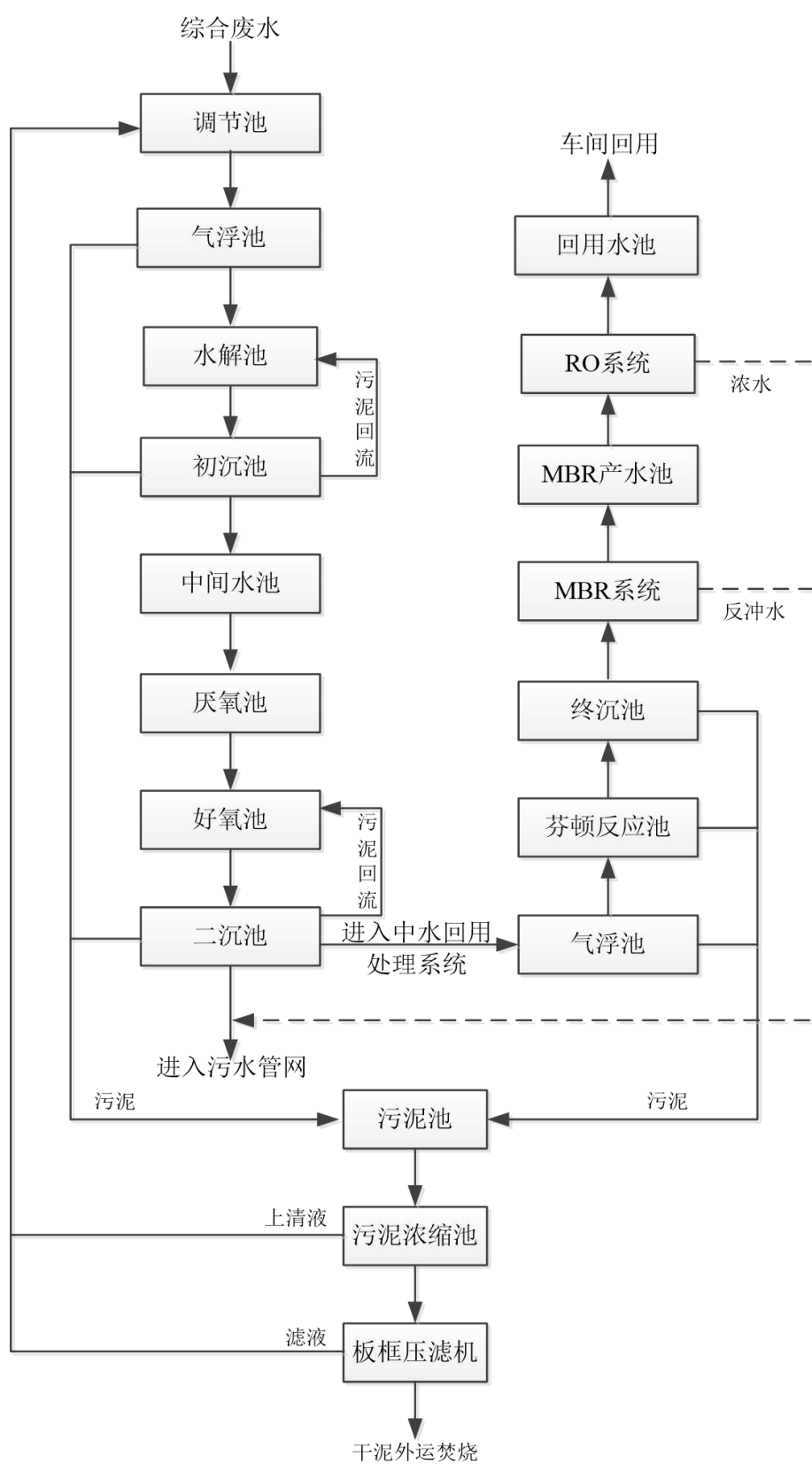
图 4.2-2 项目污水预处理及中水回用处理工艺流程图
