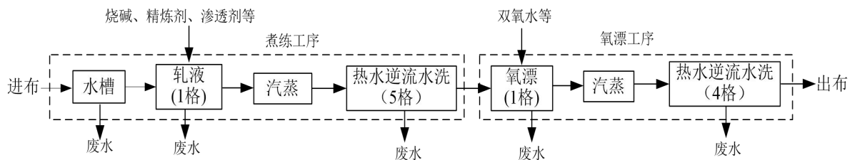
图 2.2-3 退煮漂工艺流程图
