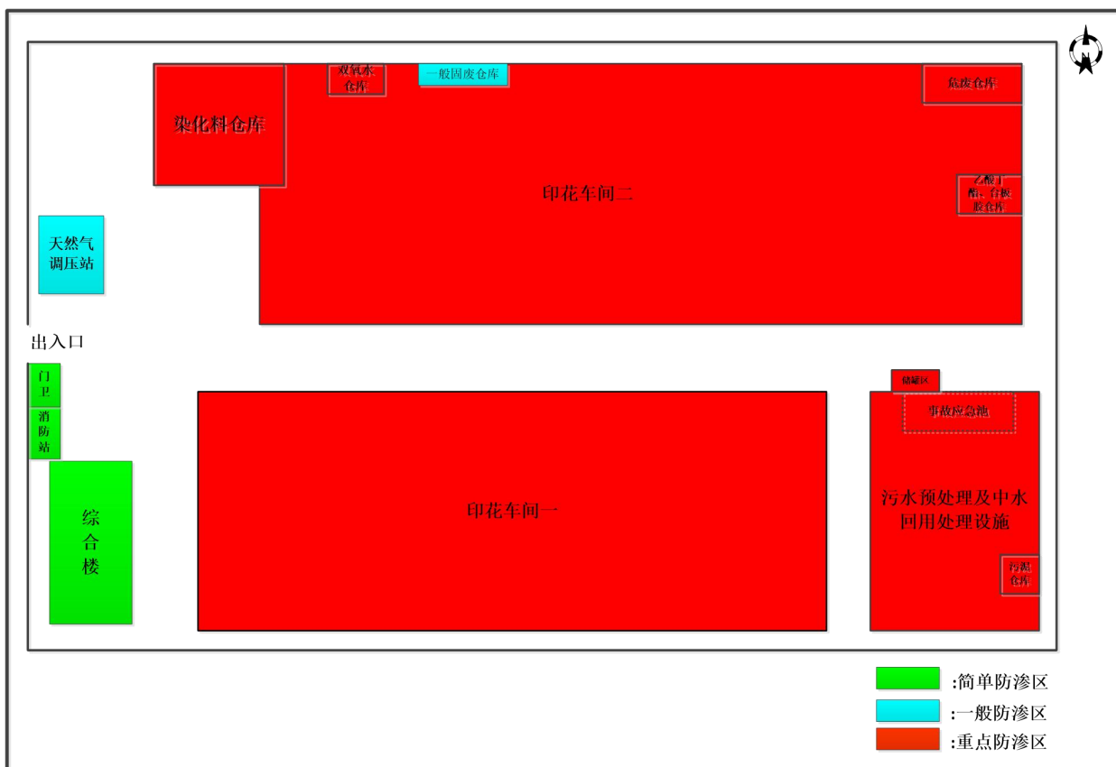
图 4.5-1 厂区地下水分区防渗示意图
