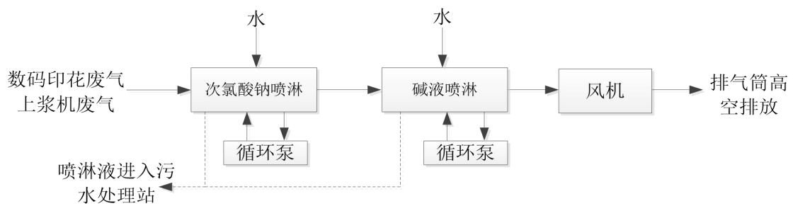
图 4.1-2 数码印花废气处理工艺流程图
