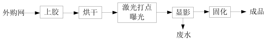
图 2.2-4 蓝光制网生产工艺流程图
