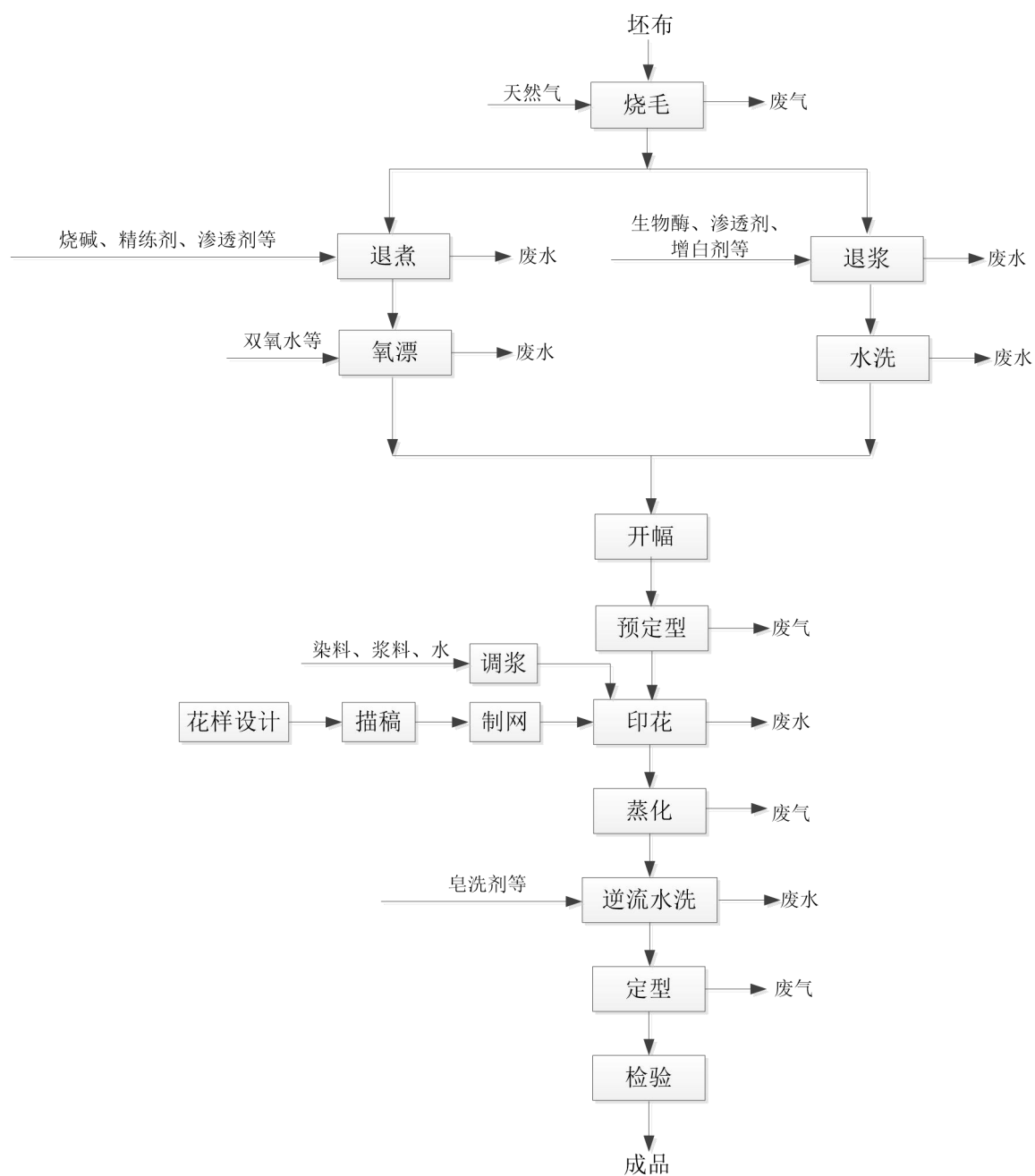
图 2.2-2 全棉机织布印花(传统印花)生产工艺流程图
