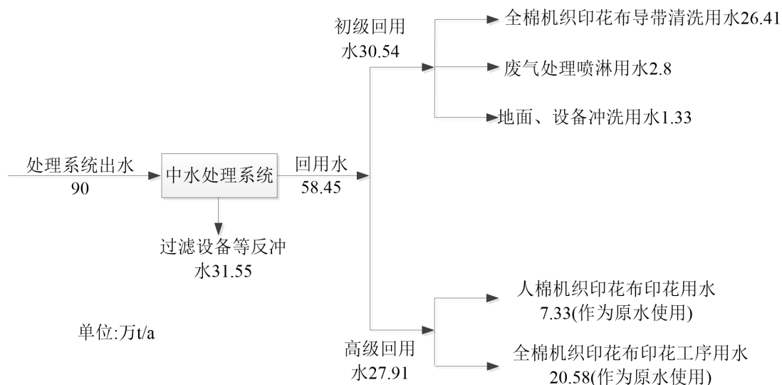
图 2.1-2 项目中水平衡图
