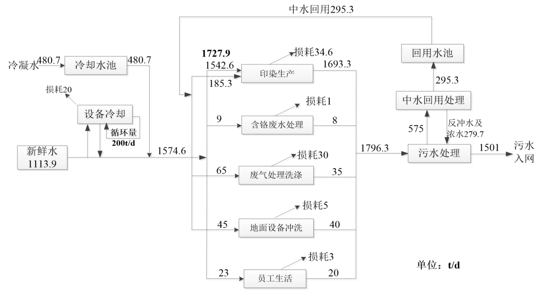
图 2.3-1 现有企业水平衡图(实际)
