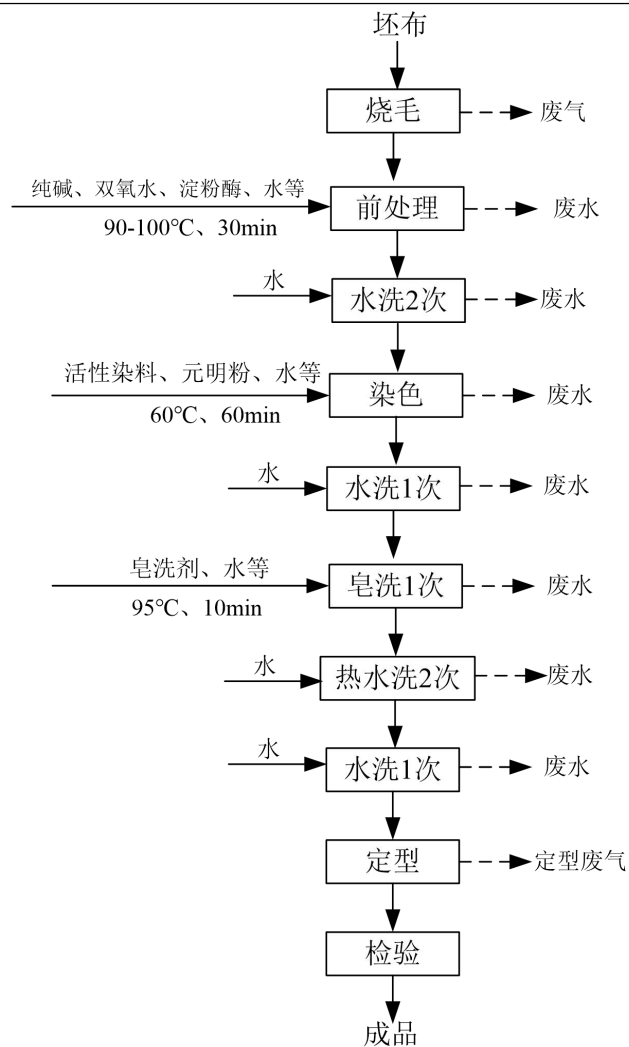
图 2.3-1 机织人棉布染色生产工艺流程图
