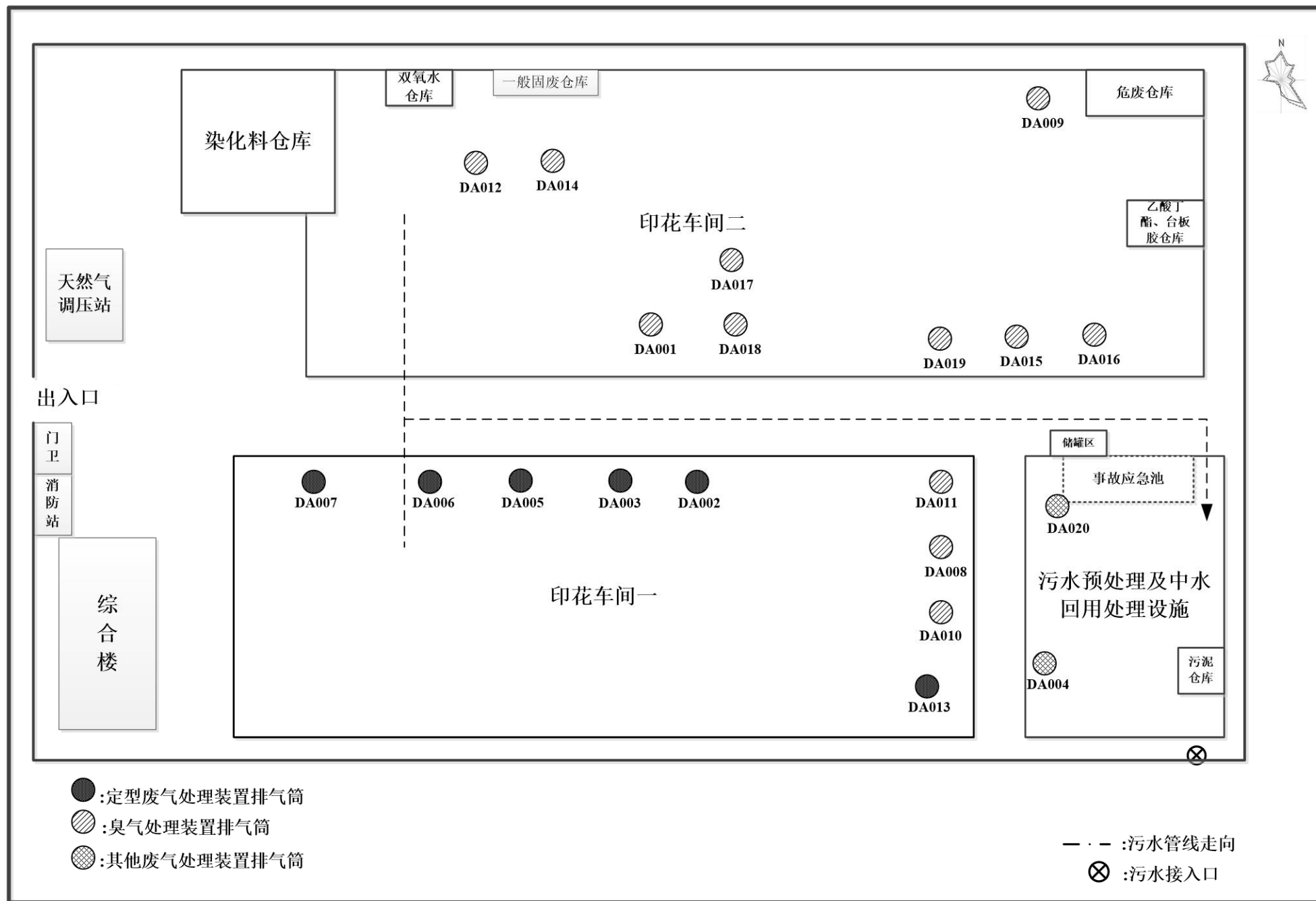
附图7 项目厂区平面布置图
