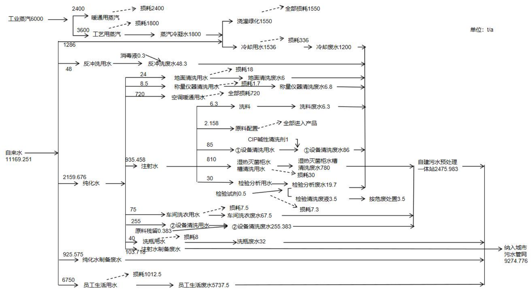
图 4-1 项目水平衡图
