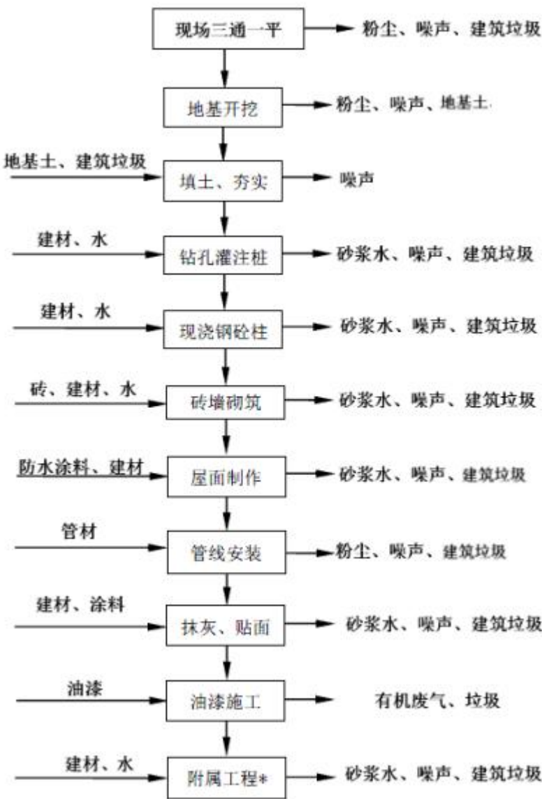
图 2-1 施工期工艺流程及排污节点图
